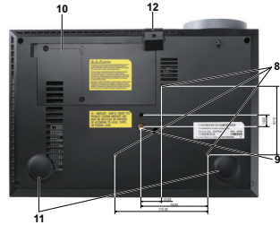
底視圖
